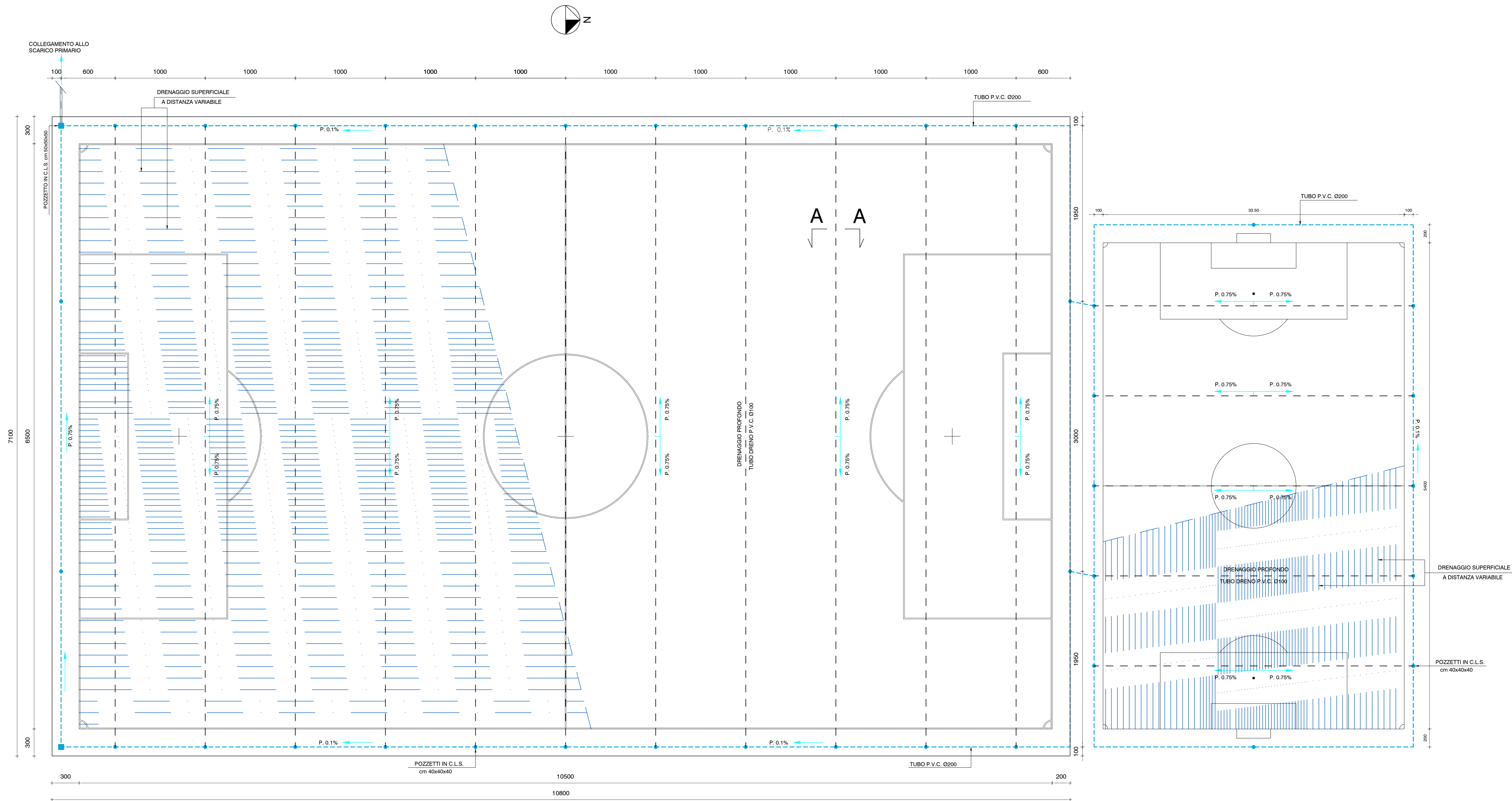
PLANIMETRIA IMPIANTO DRENAGGIO scala 1:200
