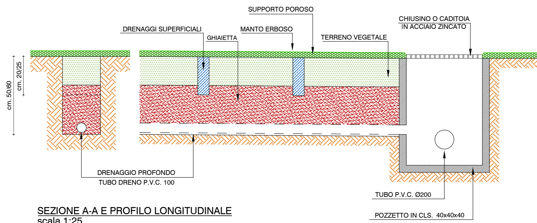
SEZIONE A-A E PROFILO LONGITUDINALE scala 1:25
